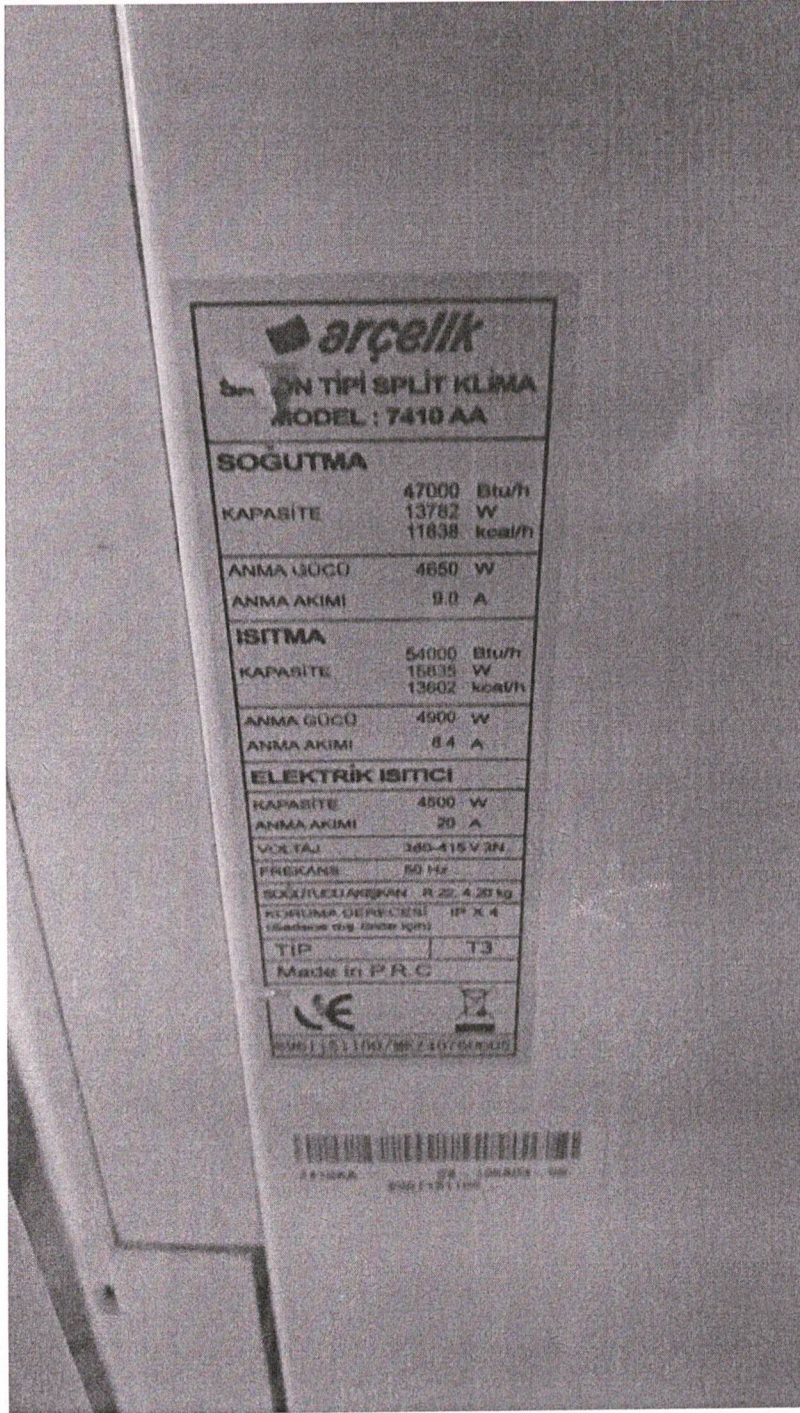
A BLOK ANA GİRİŞ SALON TİPİ KLİMA YUKARIDAKİ MARKA MODELE UYGUN İÇ ÜNİTE SERPANTİNİ(1 ADET)
